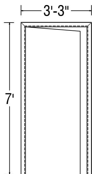
D1 3'-3" x 7'-0"
