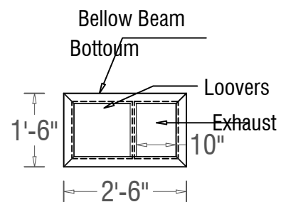
V1 1'-6" x 2'-6"
